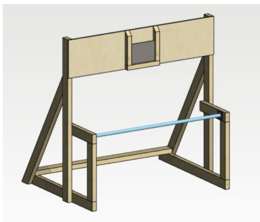
Bild 8. Knopräck KR
