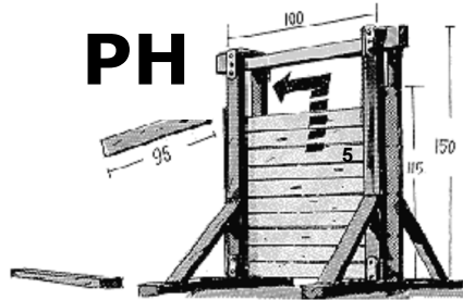
Bild 2. Plankhinder PH
